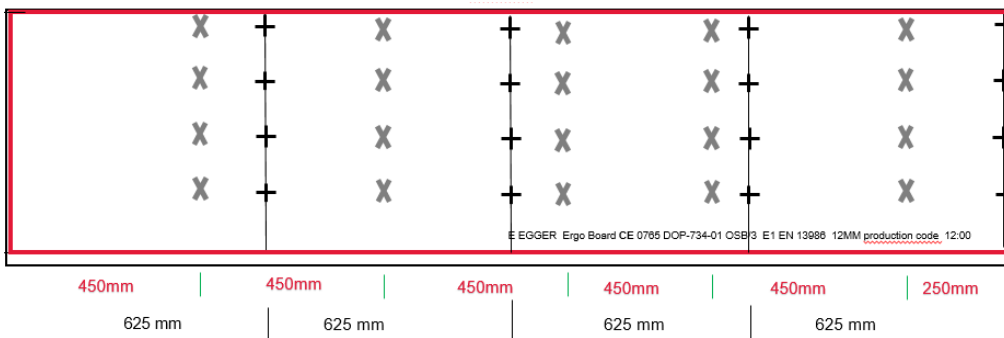
(Bild 19): Nagelrasterdruck auf der Plattenoberseite
