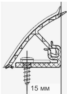
Пригвинчування основного профілю основного профілю
