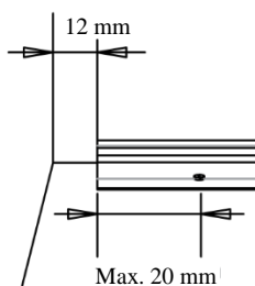
Grundprofil
