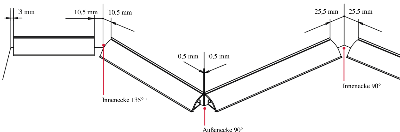
Oberprofil
