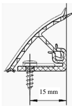
Grundprofil
