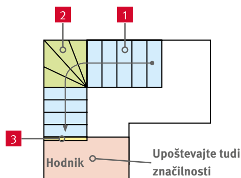
Enoramno stopnišče s podestom in pravokotno spremembo smeri
