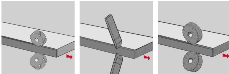
Fasen-Rundung fräsen
