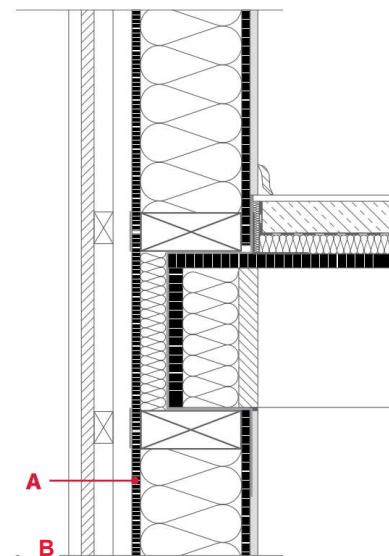
Vertikalschnitt
