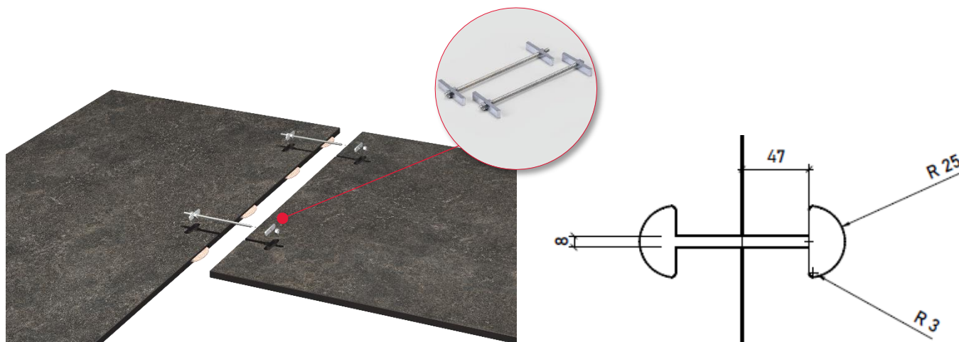
Мал. 1 З'єднання 12 міліметрових стільниць з компакт-плити Мал. 2: Схема фрезерного паза глибиною 8 мм
