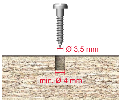
Obrázek 18: Příklad šroubu 3,5 mm
