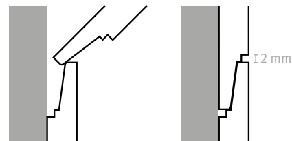
Stufenfalzprofil
