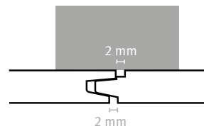
Nut- und Federprofil
