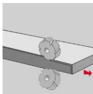
Dégrossissage : Fraise oblique (15-20°)
