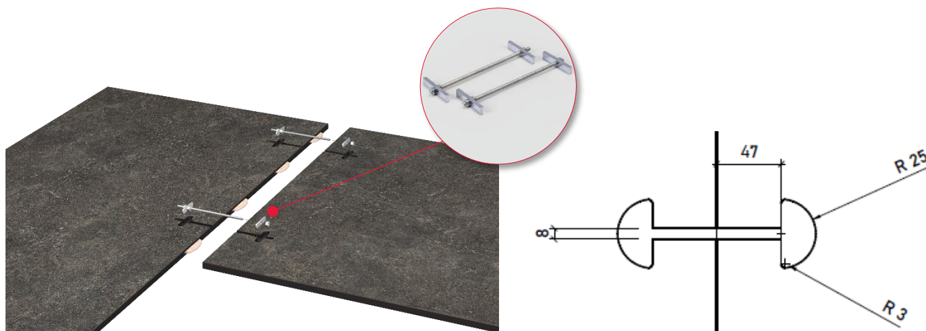
Рисунок 1: Стяжки для соединения столешниц из компакт-плиты толщиной 12 мм Рисунок 2: Схематическое изображение фрезерованной выемки под стяжку глубиной 8 мм
